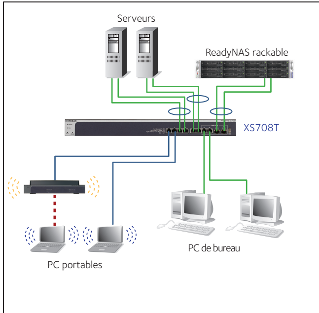
XS708T intégré dans une architecture réseau PME
