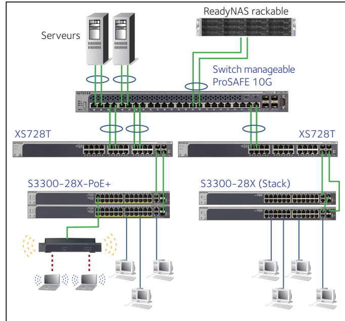
XS728T intégré dans une architecture réseau de taille moyenne
